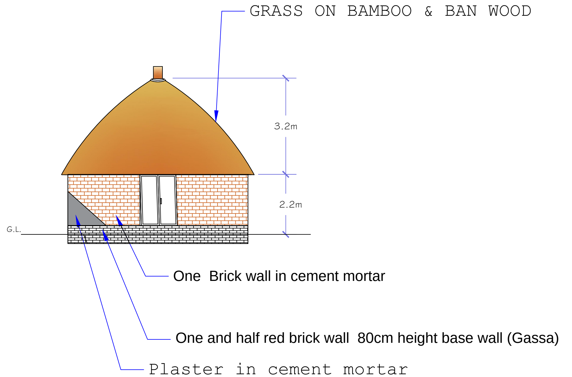
ELEVATION
